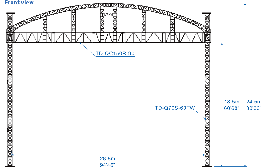
正视图 Front view
