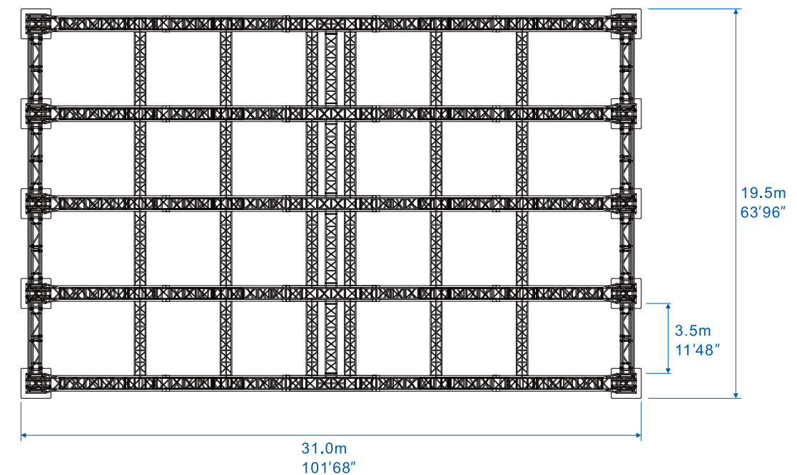
俯视图 Top view
