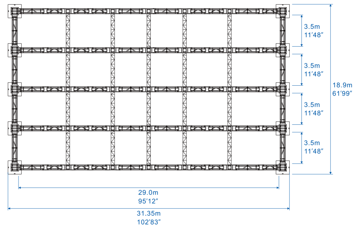
俯视图 Top view
